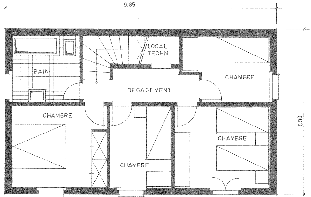
ETAGE
