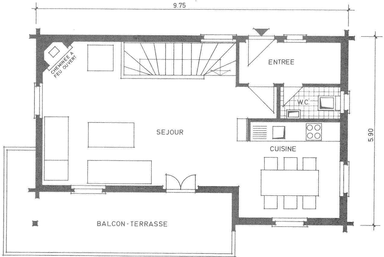
ETAGE
